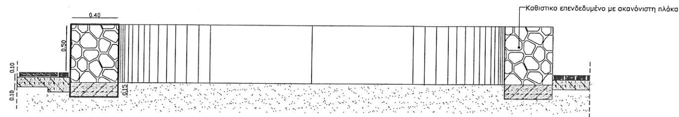
ΤΟΜΗ 1-1
